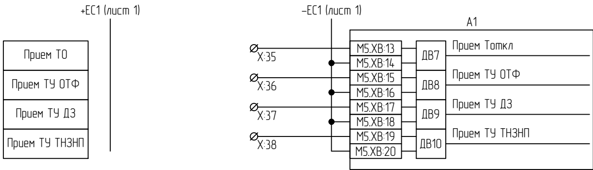
Выходные цепи
