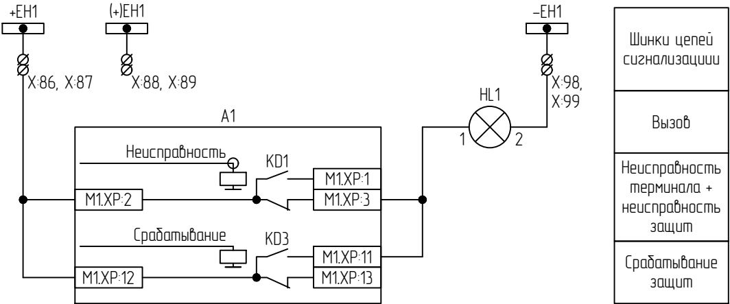
Цепи сигнализации
