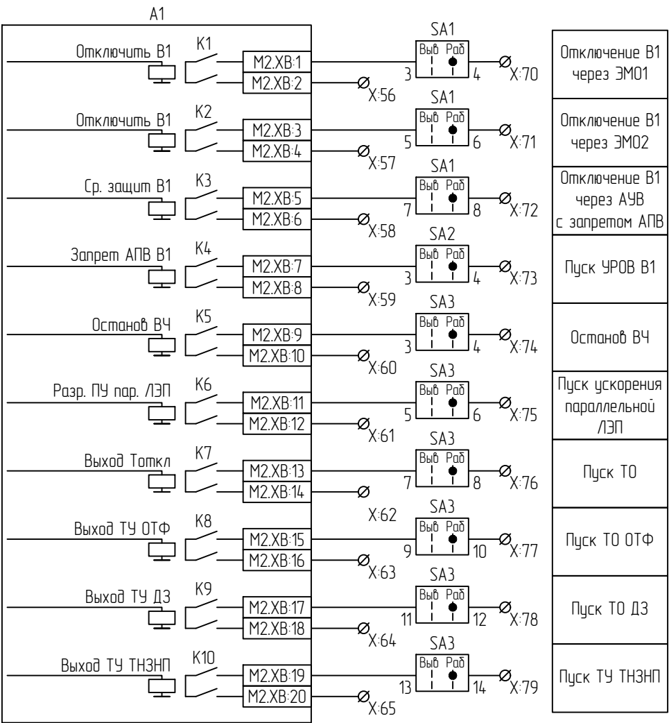
Выходные цепи
